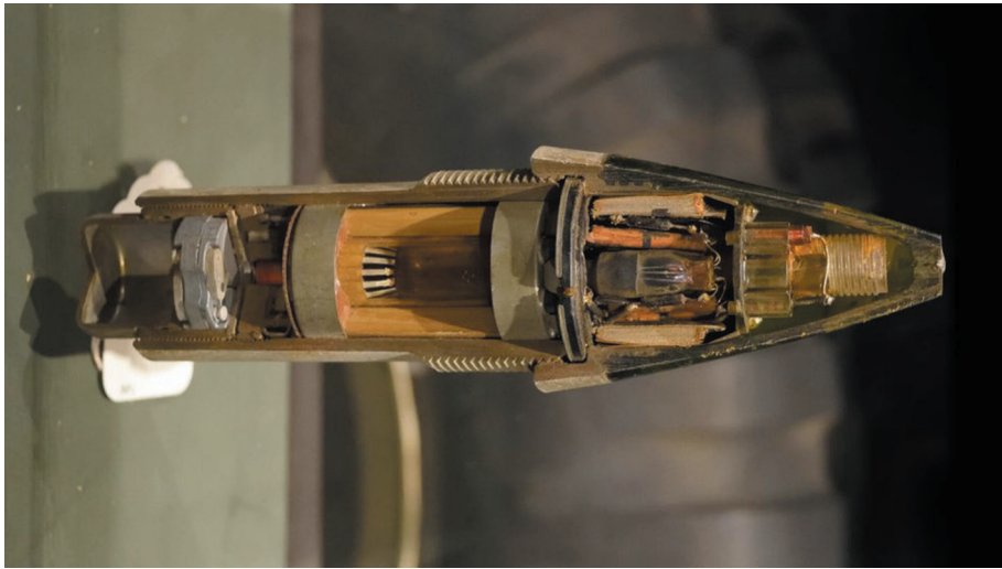
Munición de artillería americana con sensor de proximidad. (US Army)
